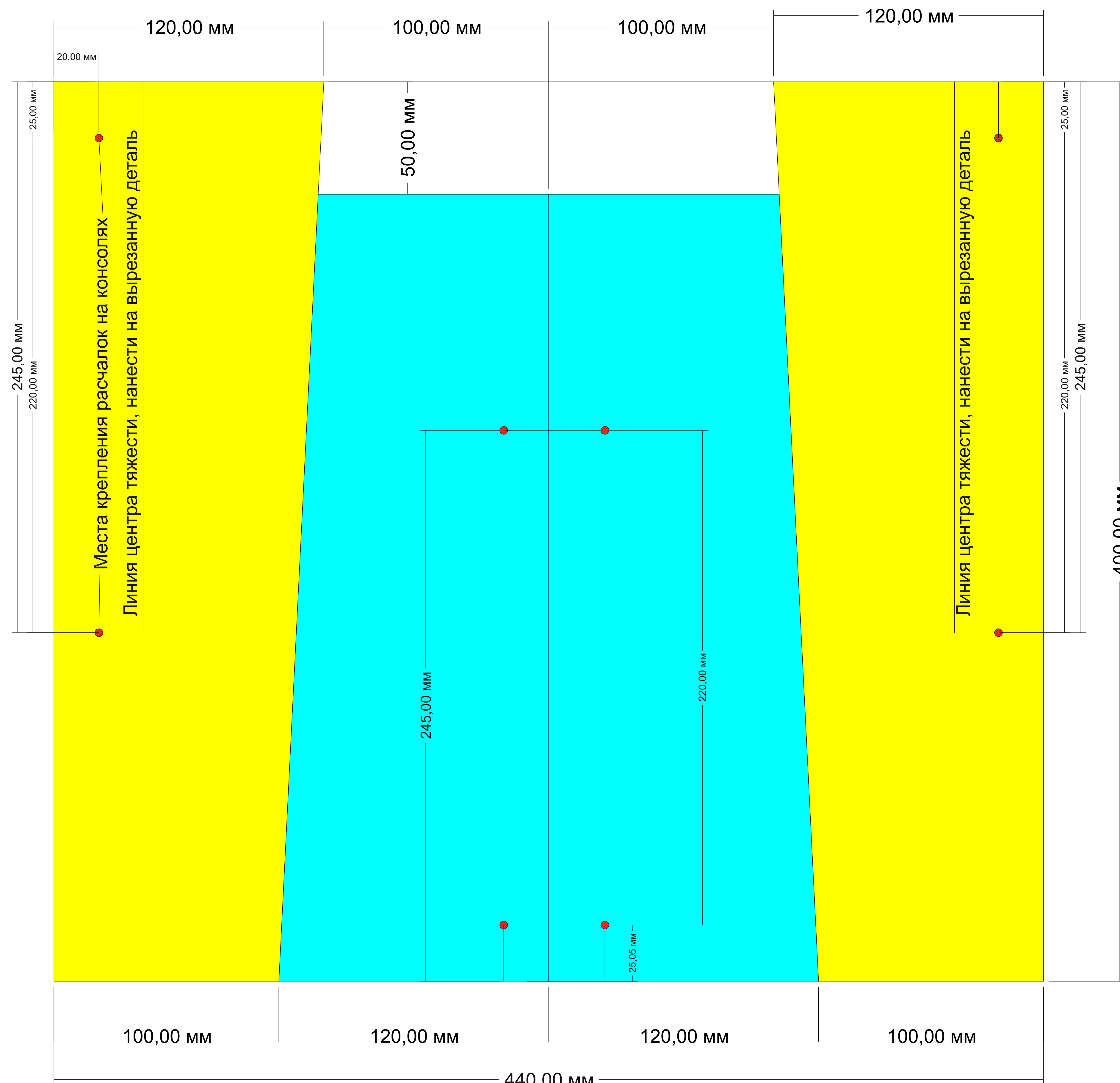
Чертежи консолей. Наносятся на лист потолочки
